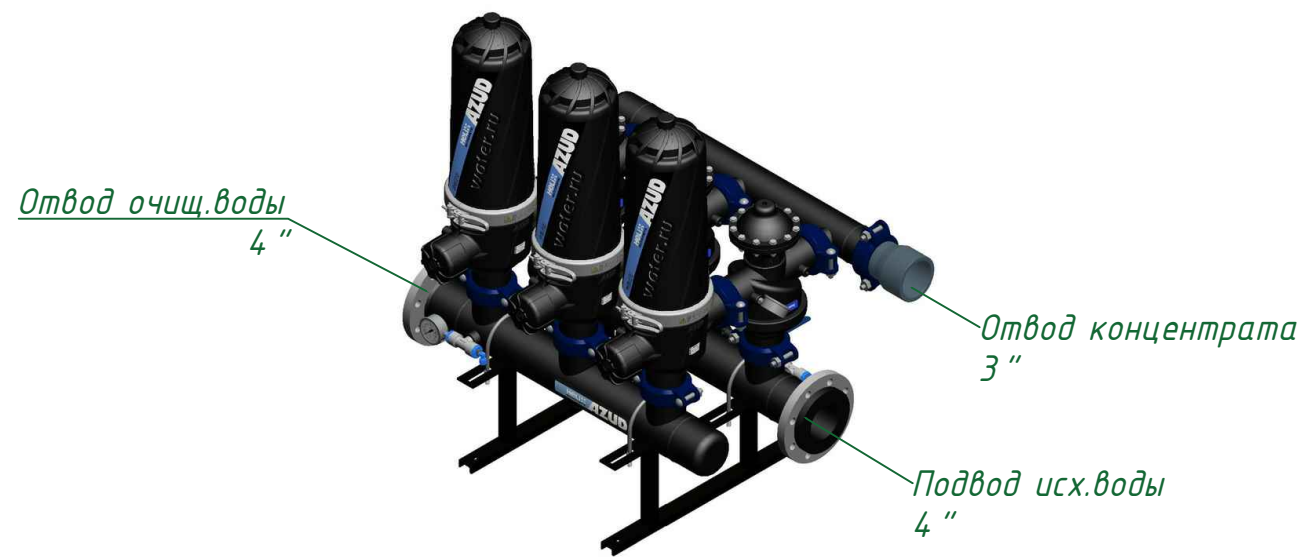
Изометрия
